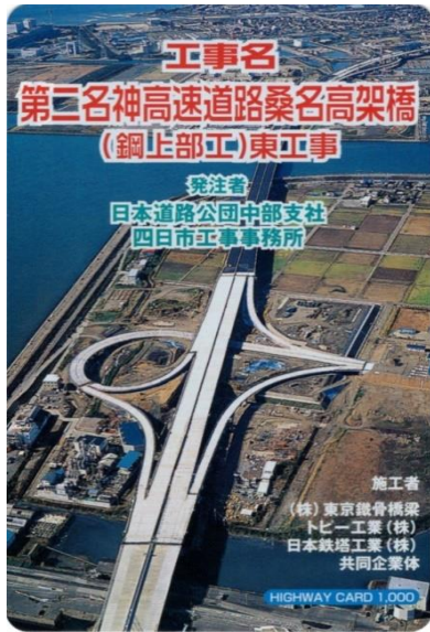
桑名高架橋(2001年竣工) 三重県桑名市
