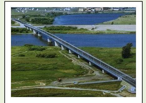
32. 砂川大橋 (1988年完成) 型式：連続箱桁 橋長：821m 所在地：砂川市・新十津川町
