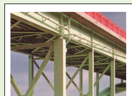
10. 原口大橋 (1978年完成) 型式：逆ローゼ桁 橋長：163.4m 所在：松前郡松前町
