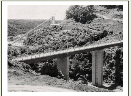
8. 川合大橋 (1976年完成) 型式：単純トラス、3径間連続鉄桁 橋長：432m 所在地：中川郡池田町
