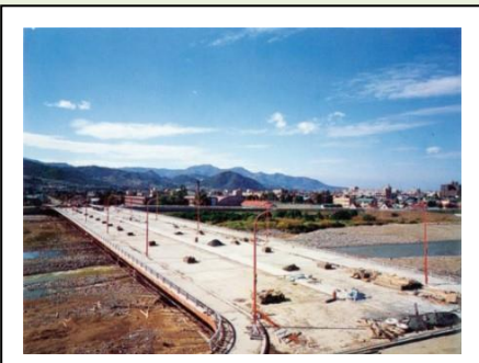
4. 南19条大橋 (1971年完成) 型式：5径間連続箱桁 橋長：236m 所在地：札幌市
