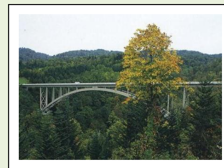
30. ウルベシ橋 (1988年完成) 型式：逆ローゼ桁・単純合成钣桁 橋長：255m 所在地：川郡美深町
