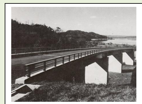
9. シラルトロ橋 (1977年完成) 型式：3径間連続鉄桁 橋長：175.5m 所在地：川上郡標茶町
