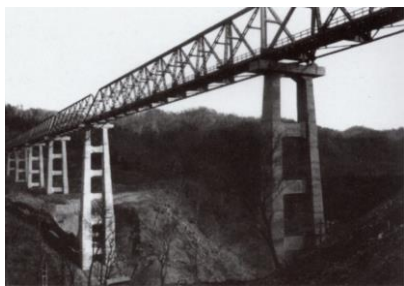
1. 三弦橋 (1958年完成) 型式：トラス橋 全長：381.6m 所在地：夕張市
