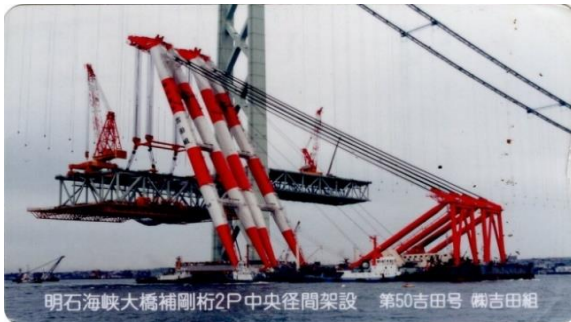
明石海峡大橋(補剛桁2P中央径間) (1998年竣工)
